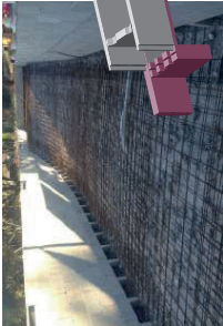
3 - Alphabloc® associé aux blocs de coffrage enduits + ferrailage.
