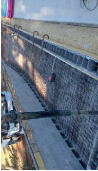
4 - Coulage du radier et des murs en une seule opération.
