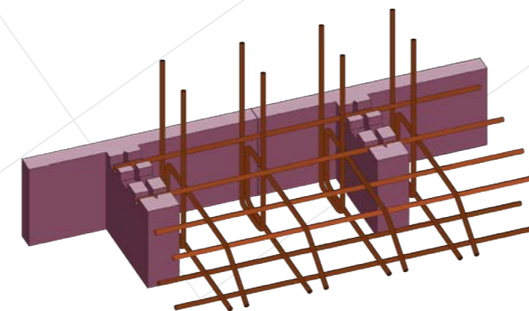
3 - Alphabloc associé aux blocs de coffrage enduits + ferrailage
